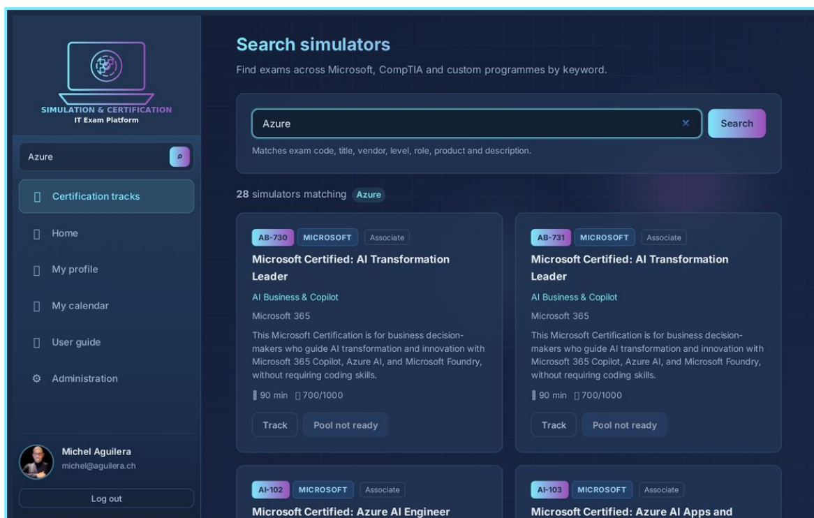
Abbildung — Simulator-Suche (Seitenleiste und Ergebnisse)
